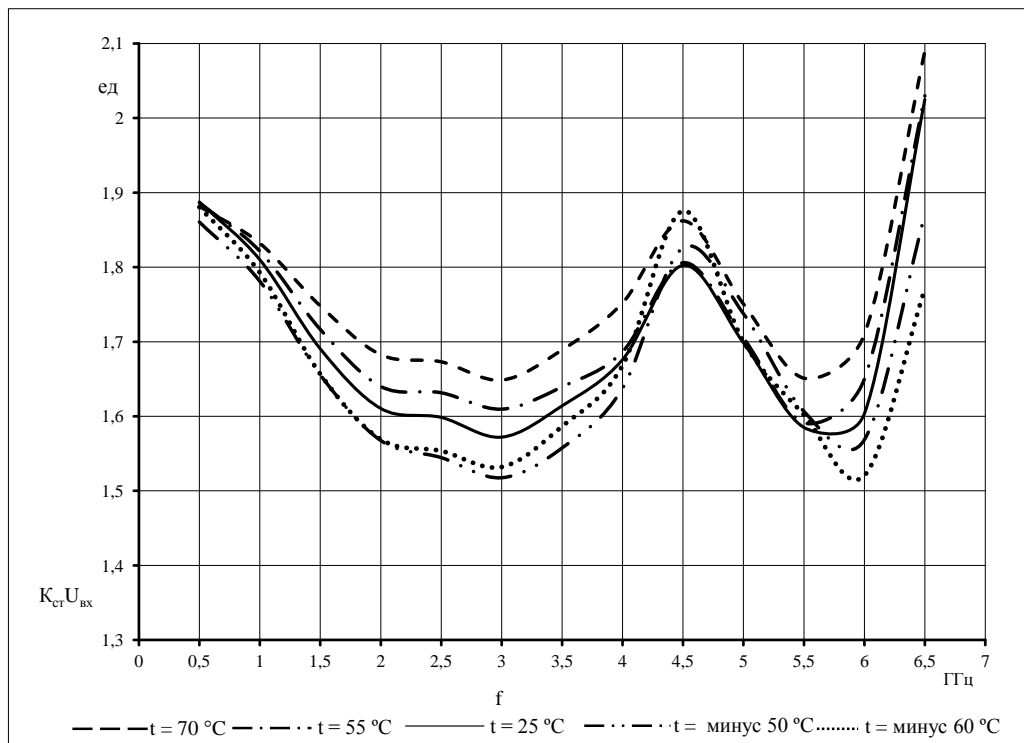
Типовая частотная зависимость K_{ст}U_{вх} в диапазоне температур
