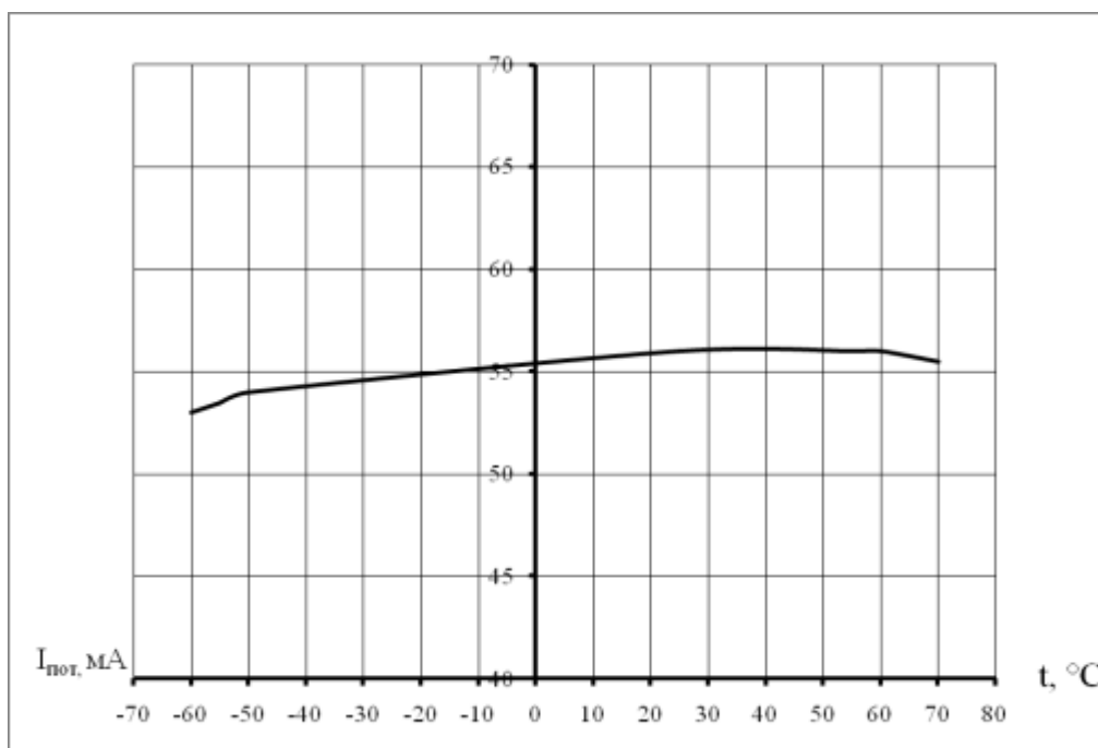
Типовая зависимость I_{пот} в диапазоне температур
