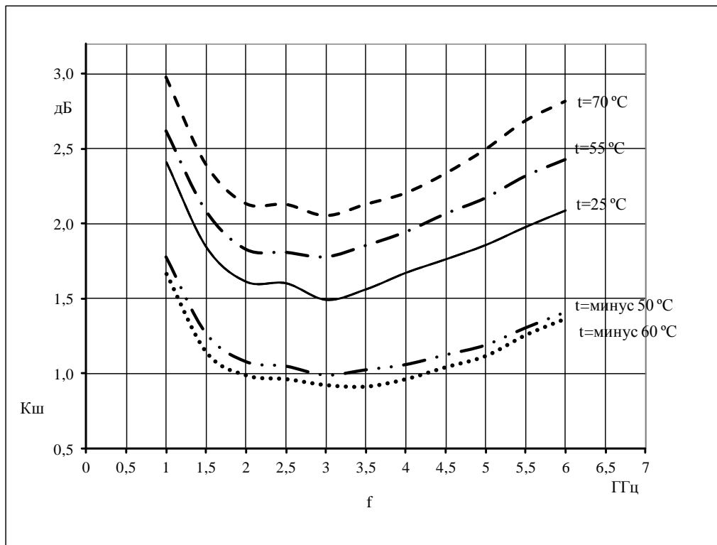
Типовая частотная зависимость коэффициента шума модуля М421443 в диапазоне температур
