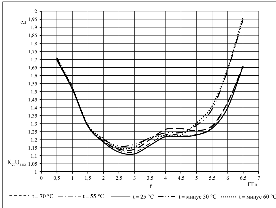
Типовая частотная зависимость K_{ст}U_{вых} в диапазоне температур
