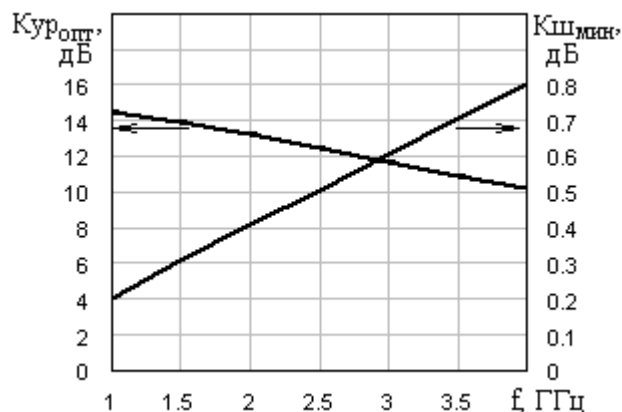
Зависимость K_{ш\ мин} и K_{ур\ опт} от частоты при U_{си}=3\ В , I_c=20\ мА
