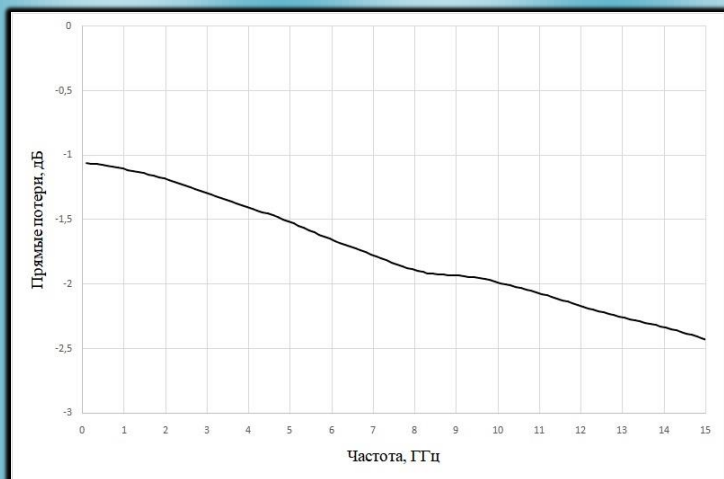
Зависимость прямых потерь от частоты
