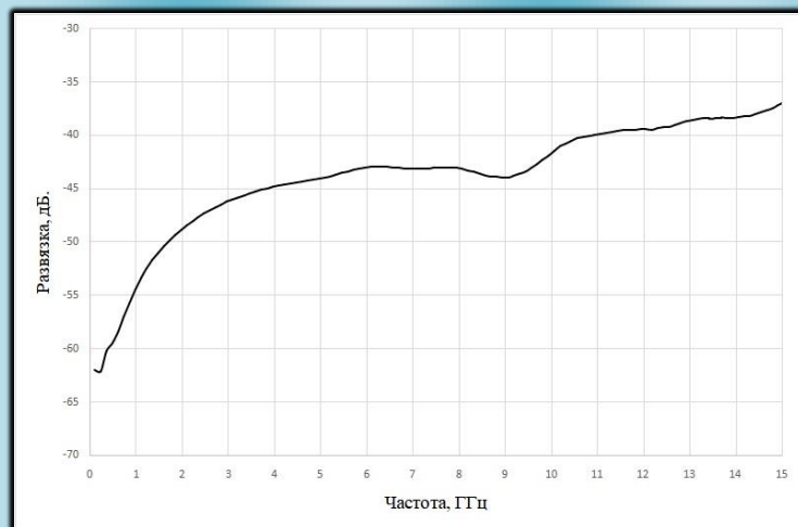
Зависимость развязки между каналами от частоты
